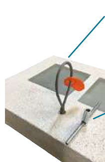
Douille de levage incorporées à la fabrication du panneau Lifting Socket and Lifting Ring
