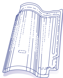
70881 N° 91 – DCL 91 GUIRAUD 31,5 x 49,5 cm – 6,3 kg 10 /m 2 Tuilier/ Tile maker DCL 91 (TERREAL COLOMIERS)
